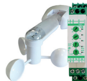
Art. 336100 Grenzwertschalter Wind Sensor inkl. Grenzwertschalter
