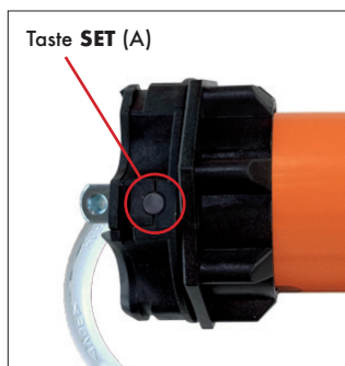
Abb.4: Detailansicht Motorkopf
