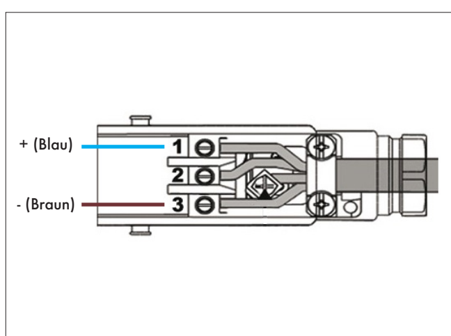
Abb.2: Anschlusskizze Lamella Statura Electronic-12V
