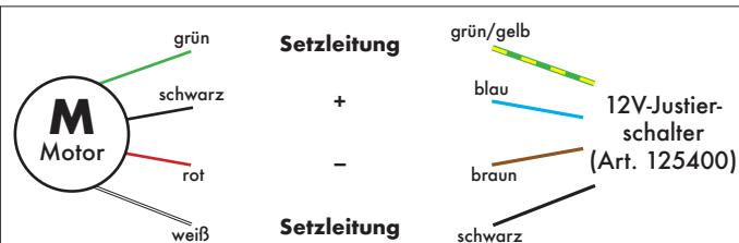
Abb.2: Anschluss Serie Electronic BL
