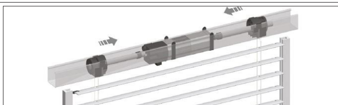
Abb.3: Einbausituation: Mittelmotoren
