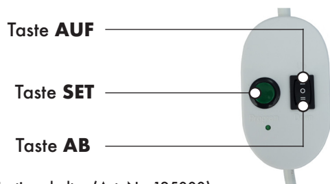
Abb. 4: Justierschalter (Art.-Nr. 125000)
