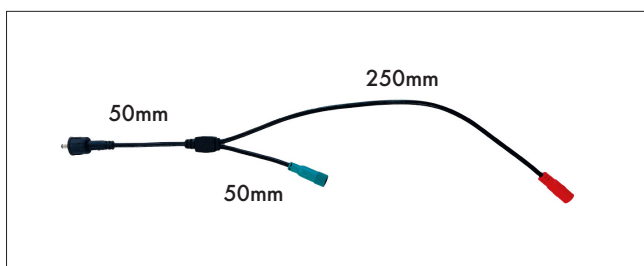
Abb. 1: Y-Connector-Kabel mit Kabellängen
