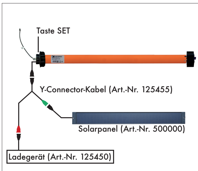
Abb. 2: Anschlussbeispiel mit Easyline Funkmotor & Steckernetzgerät
