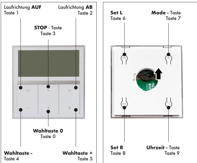
Abb.1: Vorderseite Art. 137350
